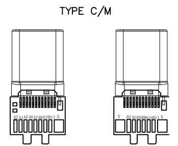
TYPE C3.1 公头焊接面
